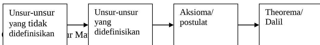
Gambar 1 Struktur Matematika
